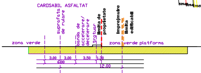
PROFIL DRUM CAROSABIL ADIACENT AMPLASAMENTULUI - DJ 121 B SECTIUNE A - A
